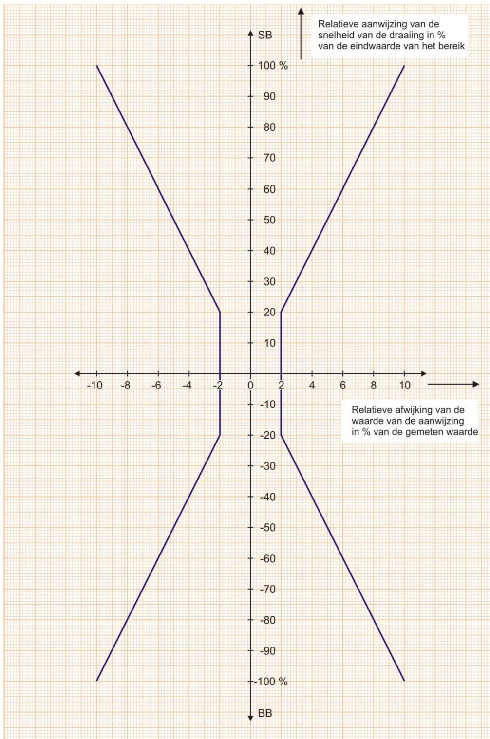
Aanhangsel Figuur 1: Tolerantiegrenzen voor bochtaanwijzers
