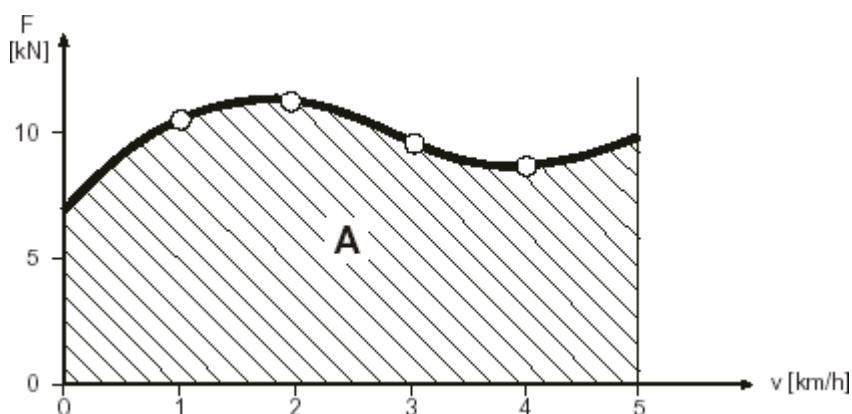
Model remkrachtschema (Bepaling van de oppervlakten AA en AB )
