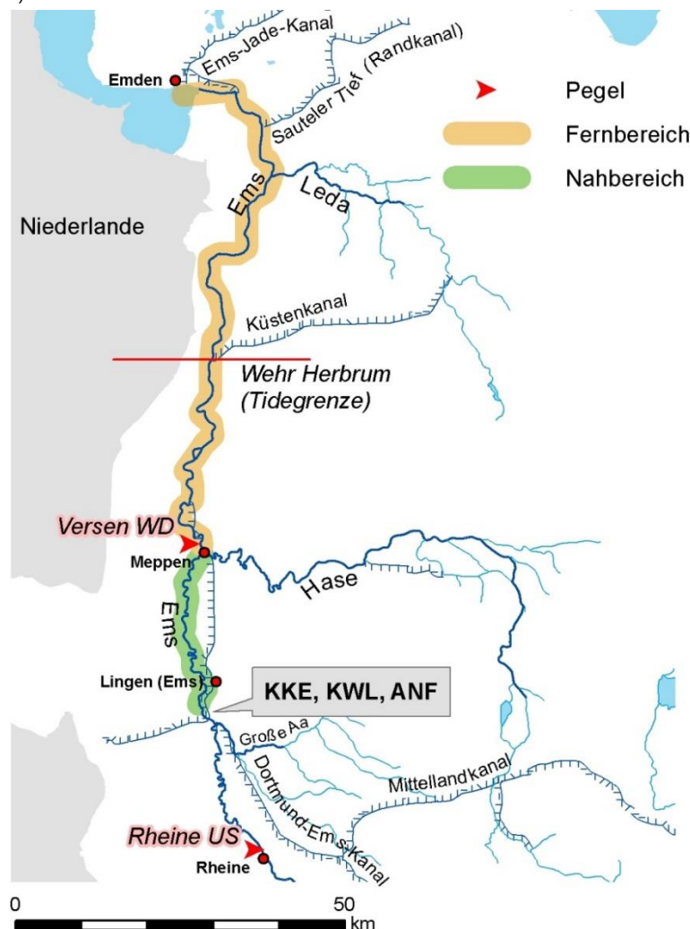
Afbeelding 1.4-1: Schematische weergave van de onderzochte afstandsgebieden van de KCE en de waterstanden van de Eems waarmee rekening is gehouden (KLE 2022)
