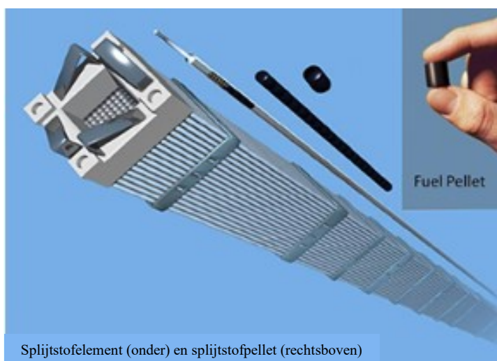
Figuur 1-5 Splijstofelement
