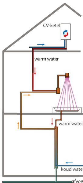
Afb. 13.4 DWTW-unit aangesloten op alleen koudepoort douchemengkraan
