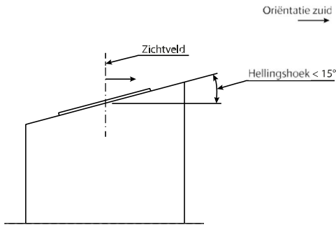
Afb. 16.2 Bijzondere situatie 1, met hellingshoek < 15°
