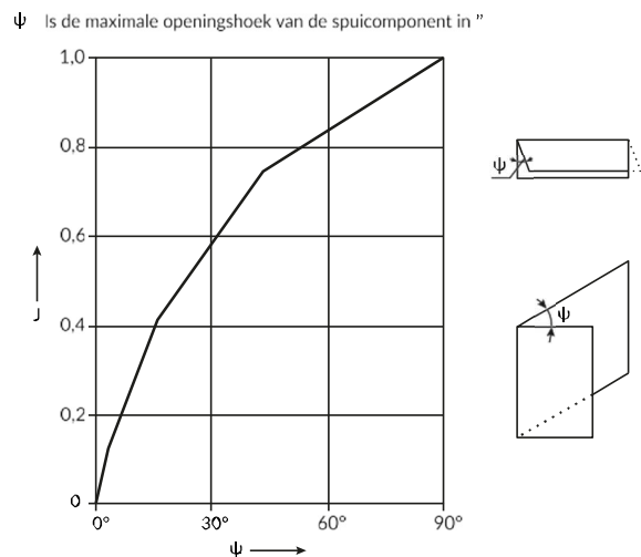
Afb. 11.4 Bepaling vermenigvuldigingsfactor J (NEN 1087)
