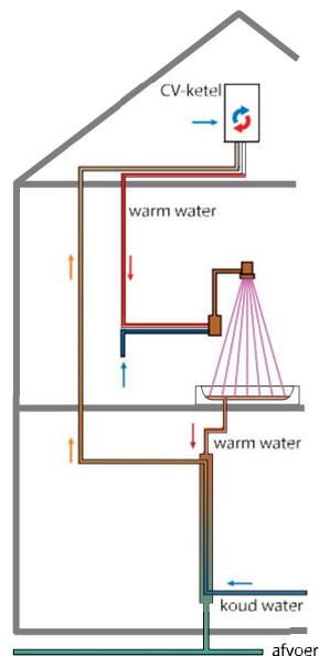
Afb. 13.5 DWTW-unit aangesloten op alleen inlaat van het toestel
