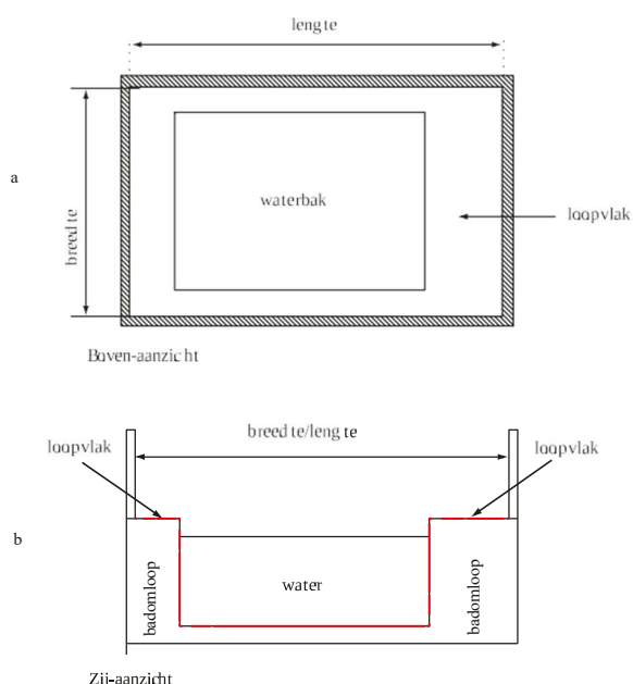
Afb. 8.5 Verliesoppervlakte zwembad, bovenaanzicht en doorsnede
