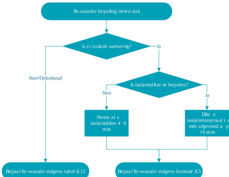
Afb. 8.16 Beslisschema voor het bepalen van de R_c -waarde van rieten-daken rieten daken en gevels
