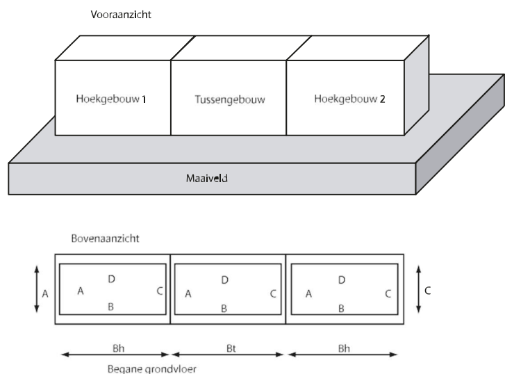
Afb. 8.6 Perimeter bij hoek- en tussengebouwen
