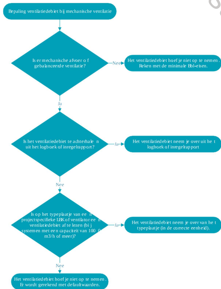
Afb. 11.1 Beslischema voor bepaling ventilatiedebiet
