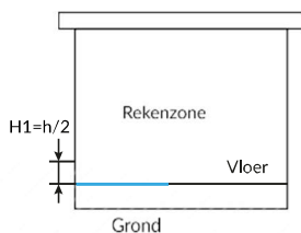
Afb. 8.10 Deel van de begane grondvloer en de buitenwand grenzend aan de grond
