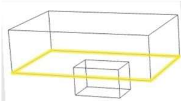
Afb. 8.8 Perimeter bij verwarmde kelder in de rekenzone (inpandig)
