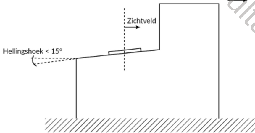
Afb. 16.3 Bijzondere situatie 2, met hellingshoek < 15°
