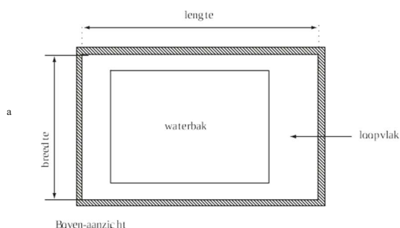
Afb. 7.8 Gebruiksoppervlakte zwembad, bovenaanzicht
