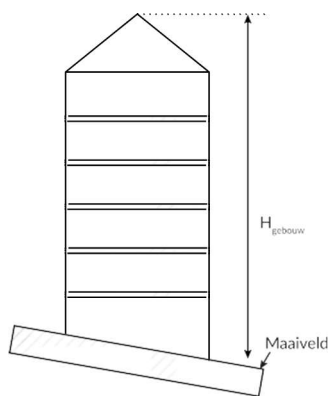
Afb. 7.4 Bepalen van de gebouwhoogte bij ongelijk maaiveld
