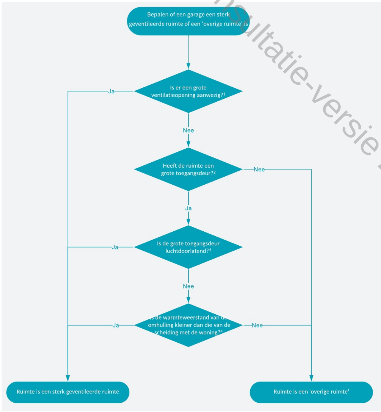
Afb. 6.x Beslisschema garages
