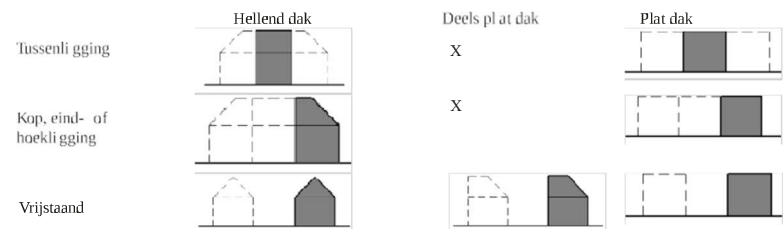
Afb. 7.2 Te bepalen gegevens dakconstructies
