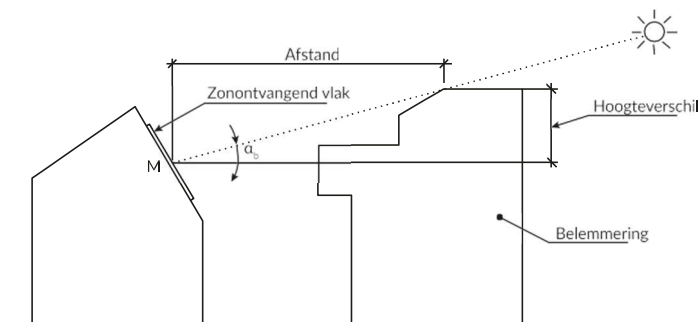
Afb. 16.4 Bepaling van de relatieve hoogte van een belemmering
