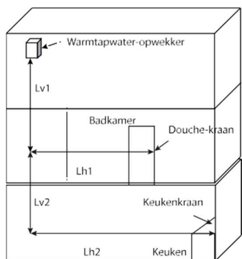
Afb. 13.1 Doorsnede vooraanzicht
