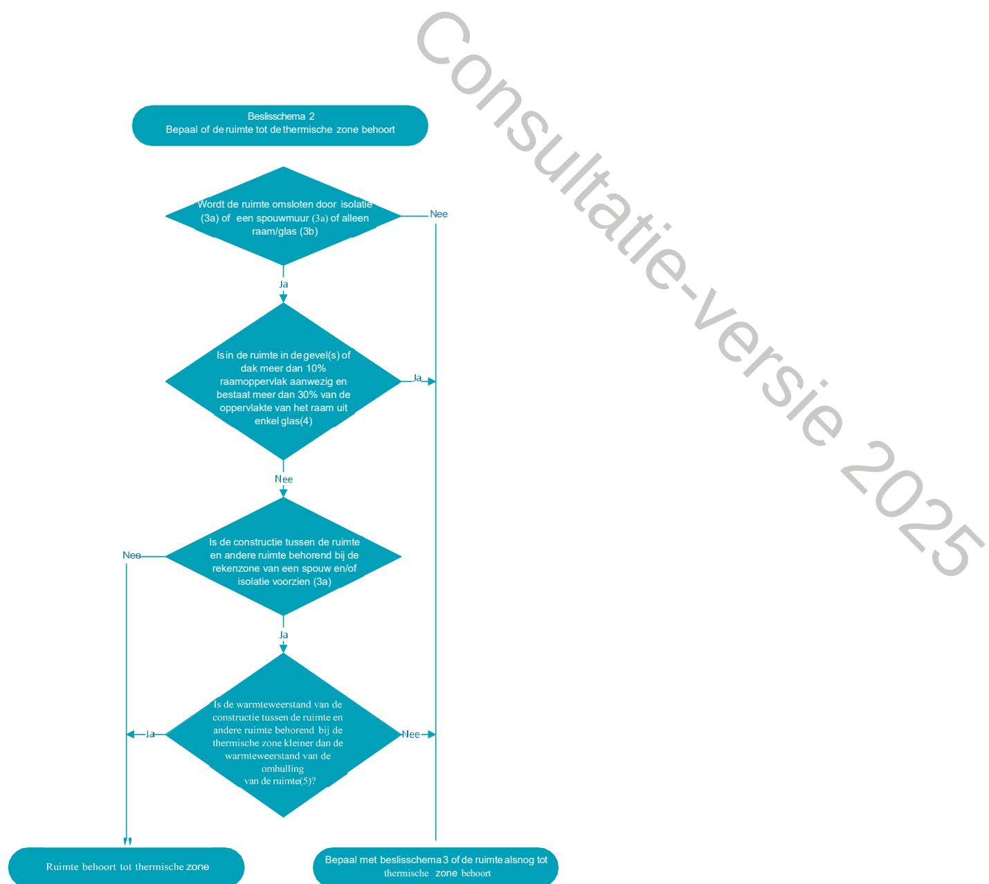
Afb. 6.2 Beslisschema 2: Thermische zone en ‘overige ruimte’
