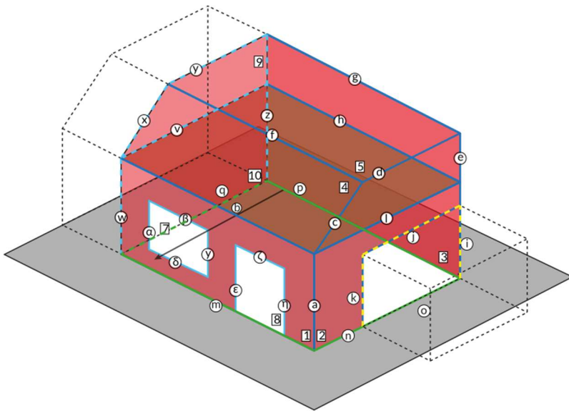
Afb. 8.13 Lineaire thermische bruggen tussen de scheidingsvlakken
