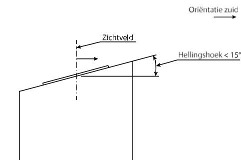
Afb. 16.2 Bijzondere situatie 1, met hellingshoek < 15^\circ
