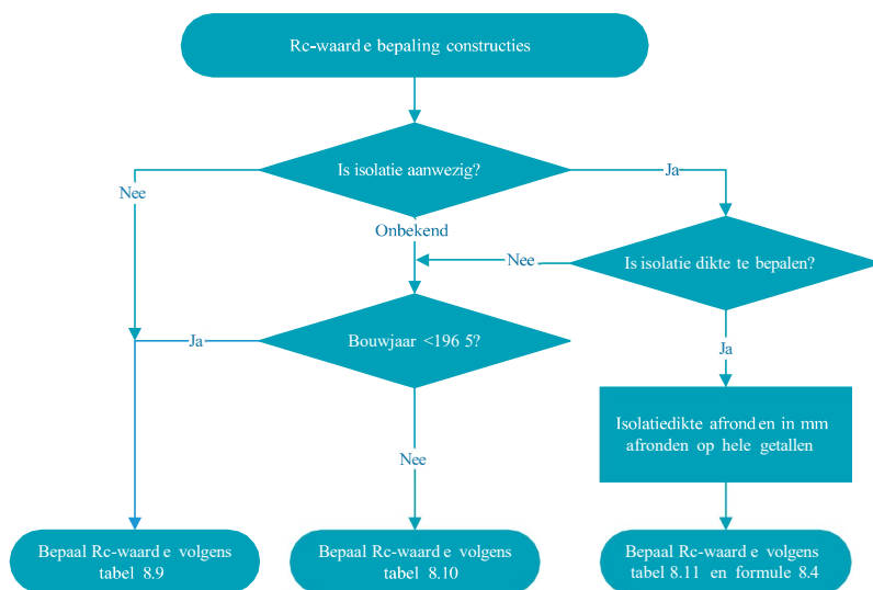
Afb. 8.15 Algemeen beslisschema voor de R_c -waarden
