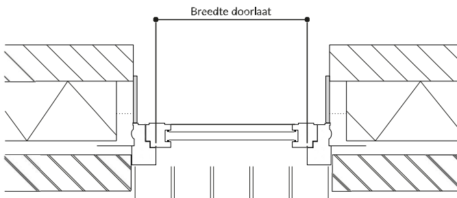
Afb. 11.3 Bruto breedte van de doorlaat (horizontale doorsnede opening)
