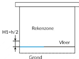
Afb. 8.10 Deel van de begane grondvloer en de buitenwand grenzend aan de grond
