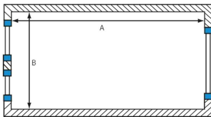
Afb. 7.6 Meten tussen de opgaande scheidingsconstructies
