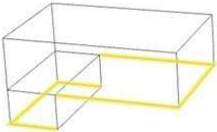
Afb. 8.7 Perimeter bij verwarmde kelder in de rekenzone
