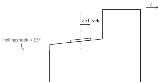
Afb. 16.3 Bijzondere situatie 2, met hellingshoek < 15^\circ
