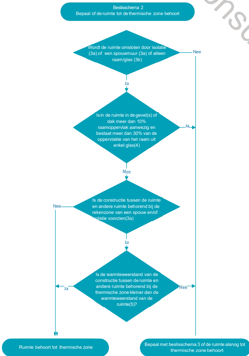
Afb. 6.2 Beslisschema 2: Thermische zone en 'overige ruimte'
