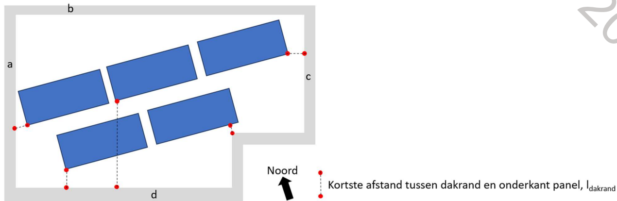
Bovenaanzicht: dak met 5 panelen en dakrand
