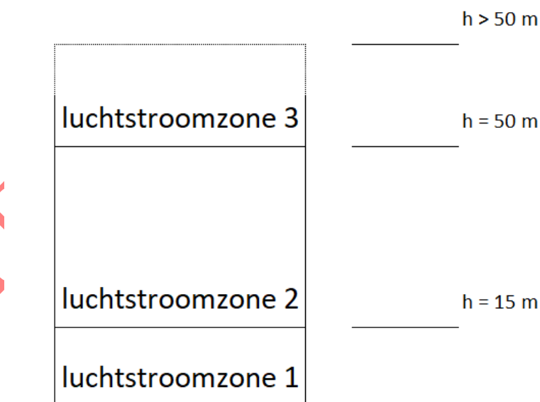
Figuur 11.2 — Toelichting luchtstroomzone
